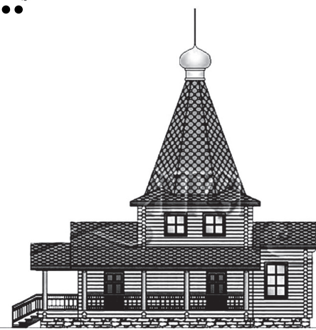
Проект "ЦЕРКОВЬ ПР-20" Общая площадь - 74,2 м 2
