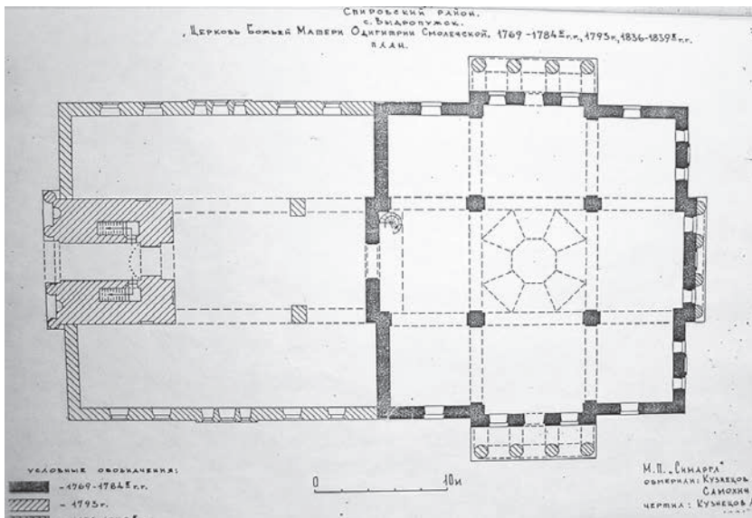
План Смоленской церкви с. Выдропужск, 1991 г. Чёрным цветом показана часть здания, построенная по проекту С.И. Чевакинского
